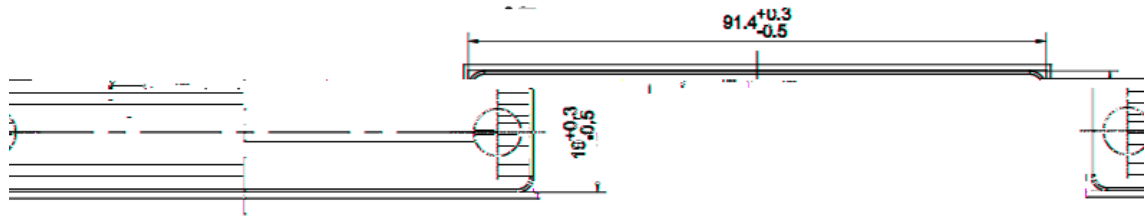
A视图
